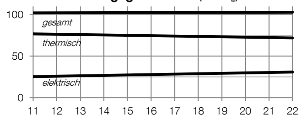
Wirkungsgradkurven [% / kW_{el} ]
