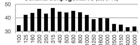
Schalldruckpegelkurve [dB(A) / Hz] 5)
