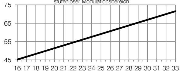
Leistungskurve [kW th / kW el ] stufenloser Modulationsbereich
