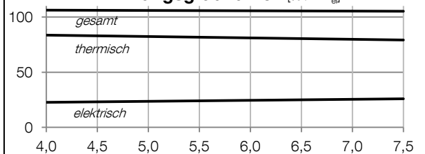
Wirkungsgradkurven [% / kW el ]
